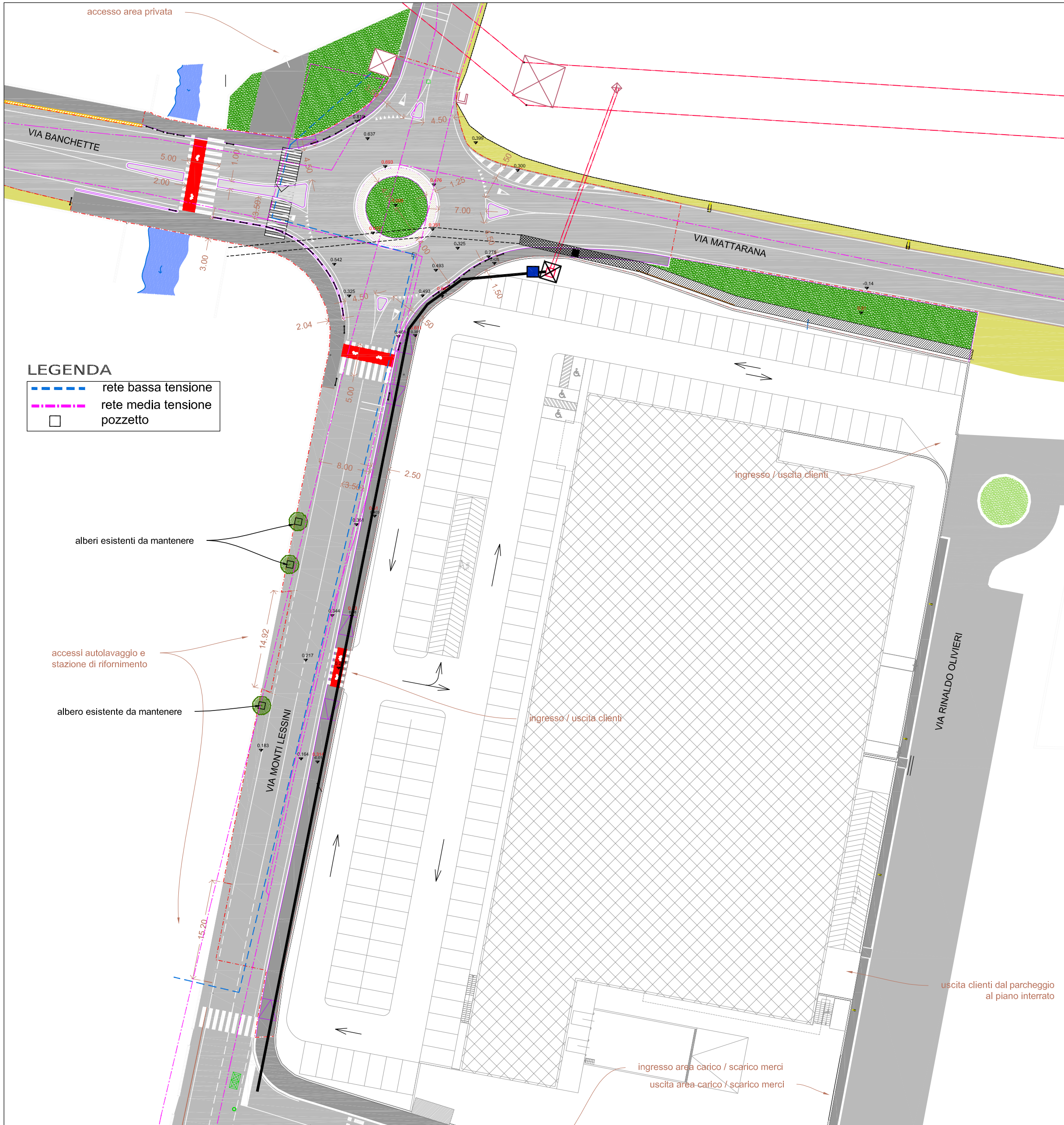
Planimetria stato di progetto con evidenziate le linee di energia elettrica esistenti scala 1:500
