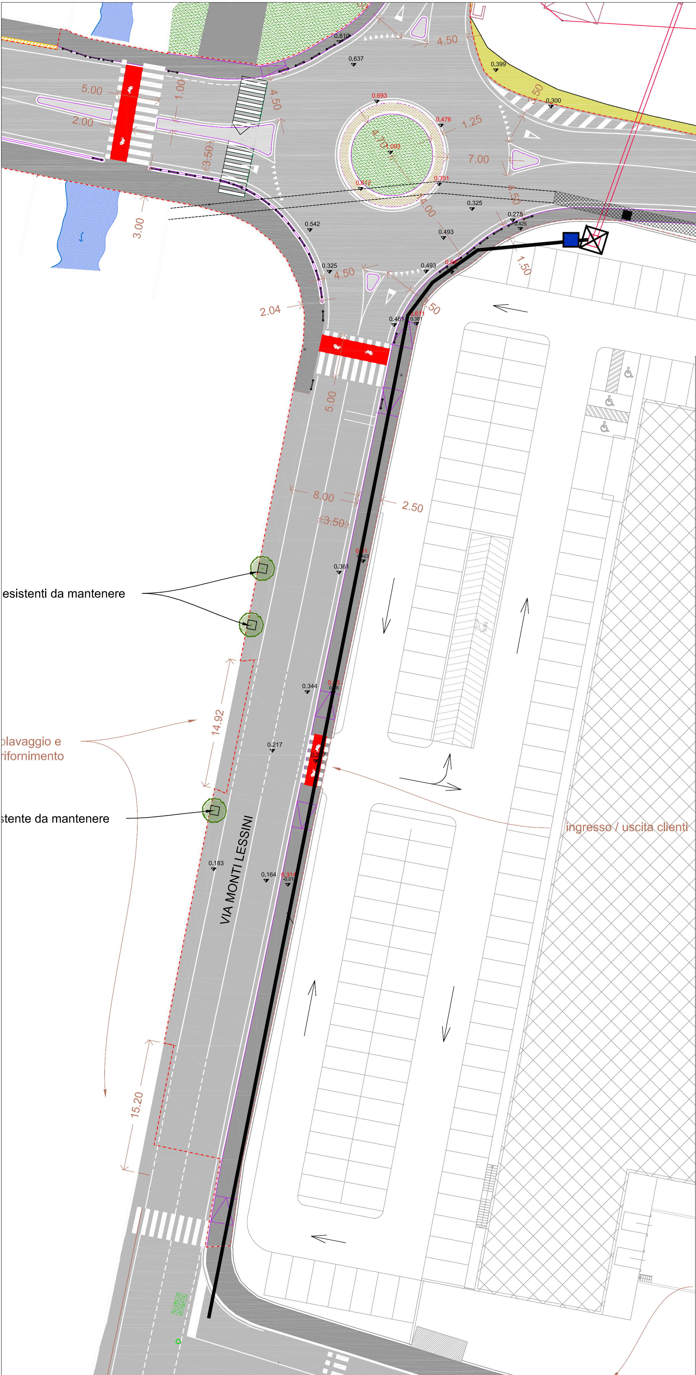
Planimetria stato di progetto rete energia elettrica scala 1:250
