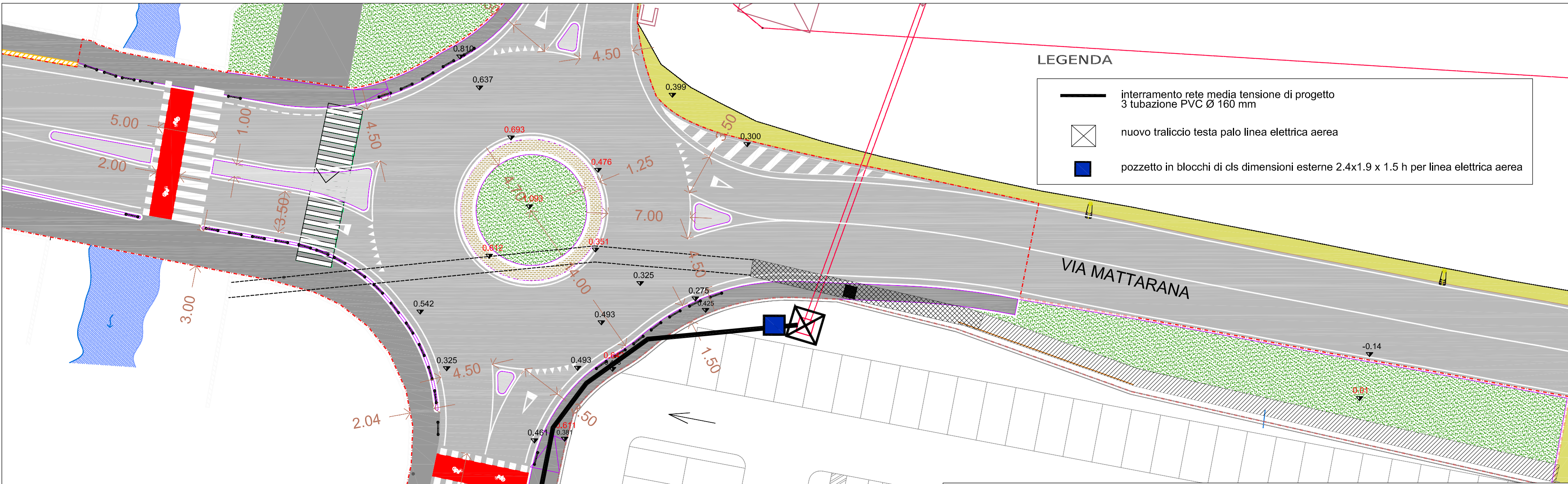
Planimetria stato di progetto rete energia elettrica scala 1:250
